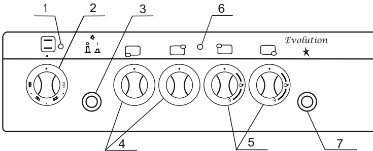
Панель управления плиты модели 506022.02гэ
